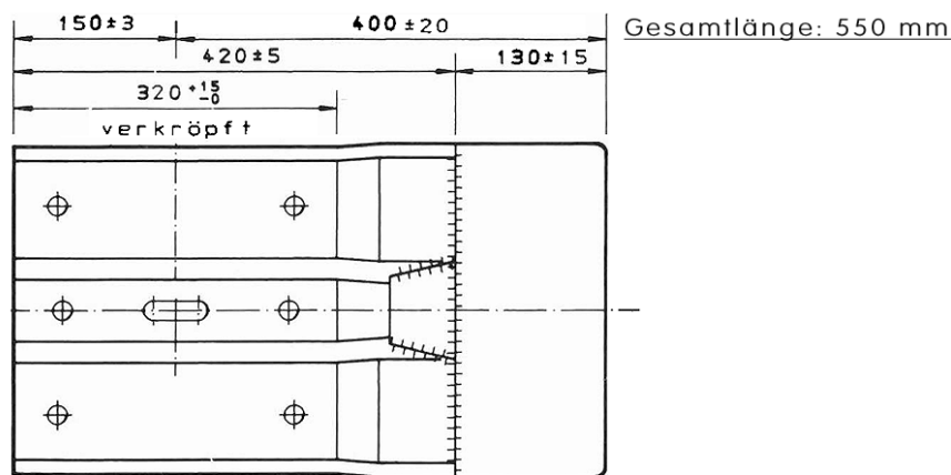
Teil Nr. 12.11 Kopfstück mit Tropflöchern
