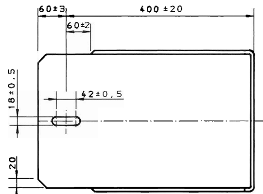
Schnitt A-A
