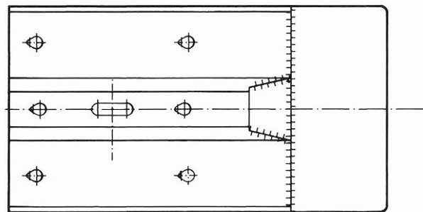
Teil Nr. 12.11 Kopfstück mit Tropflöchern
