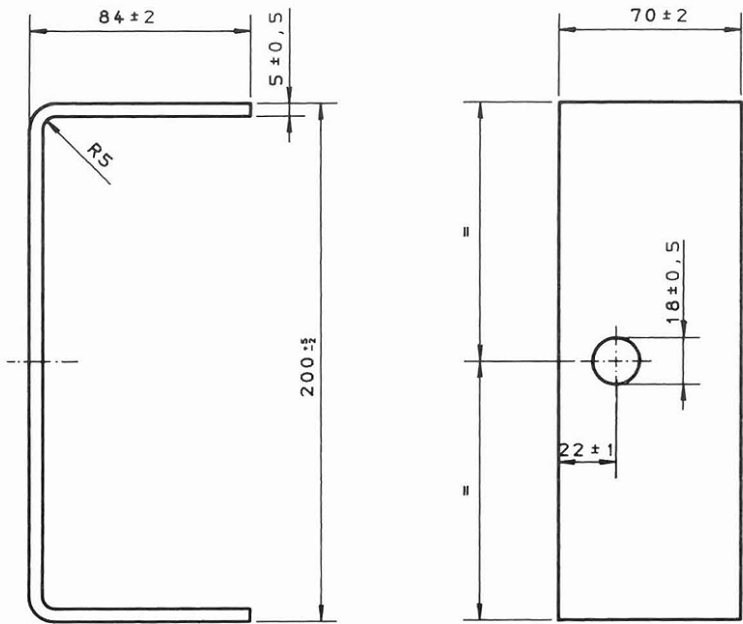
Teil Nr. 4.00 Stützbügel Profil A
