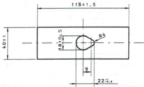
Teil Nr.10.10 Decklasche M10
