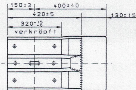
Teil Nr. 12.16 Anschlußkopfstück mit Tropflöchern
