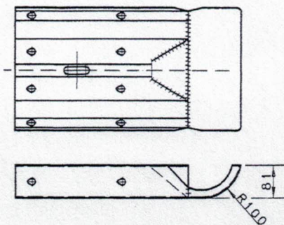
Teil Nr. 12.15 Anschlußkopfstück mit Rundlöchern
