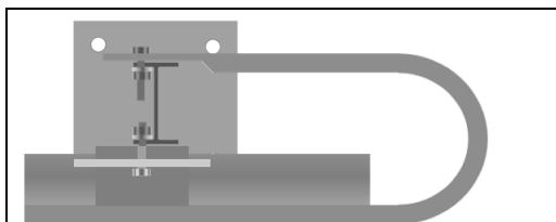
Links: Draufsicht Pfostenverschraubung mit Kopfstück
