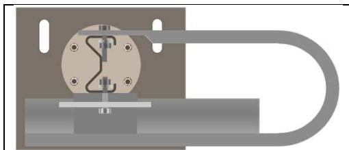
Links: Draufsicht Pfostenverschraubung mit Kopfstück
