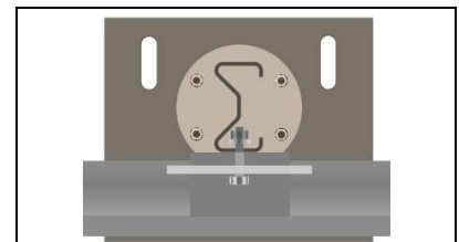
Links: Draufsicht Pfostenverschraubung mit Kopfstück
